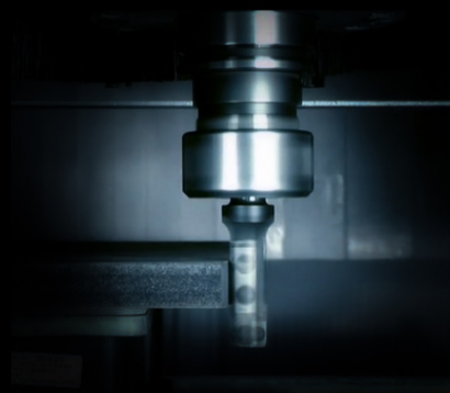
12 kW rezkar 1.000 - 24.000 obratov na minuto
