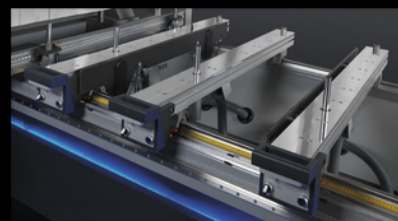
6 konzol za vakuumska prijemala
